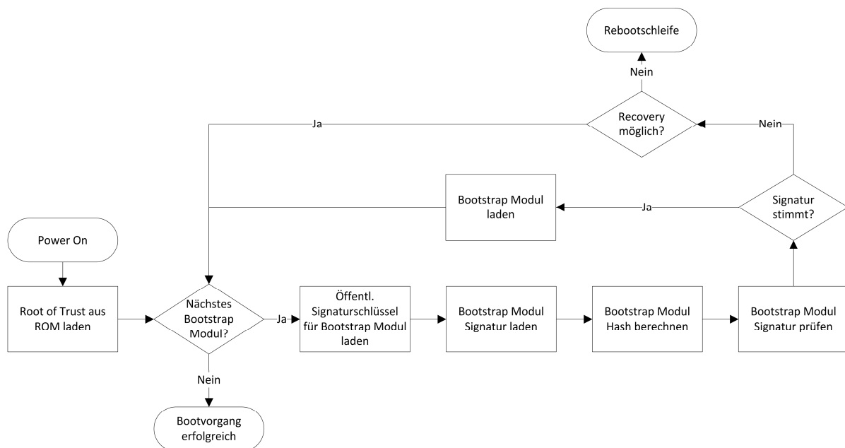
Abb. 3: Secure-Boot-Verfahren
