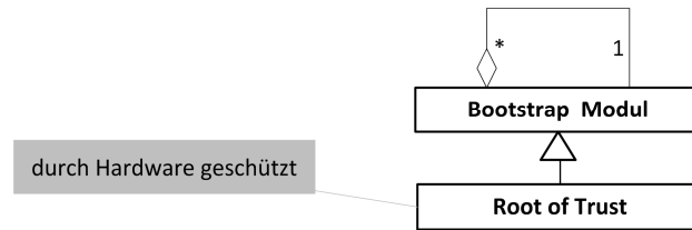
Abb. 2: Secure Boot-Pattern gem. [LSW10]
