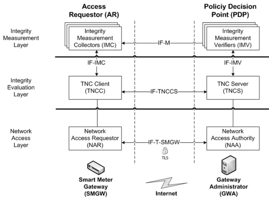
Abb. 4: TNC-Schichtenmodell mit relevanten Komponenten des Systemkonzepts
